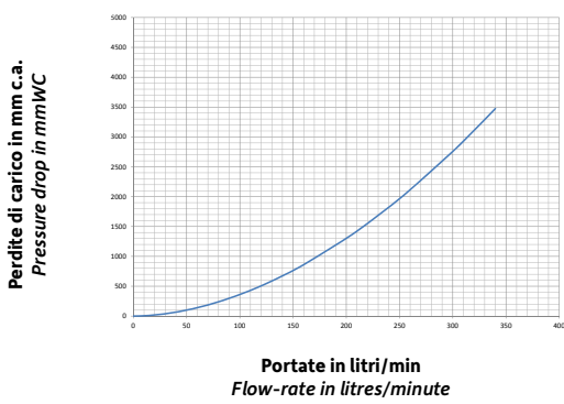
Scambiatore a fascio tubiero 5 m 2 Tube bundle heat exchanger 5 m 2
