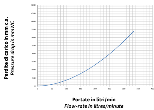
Scambiatore a fascio tubiero 4 m 2 Tube bundle heat exchanger 4 m 2
