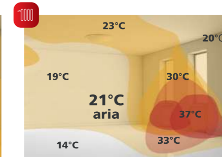
Radiatore tradizionale
